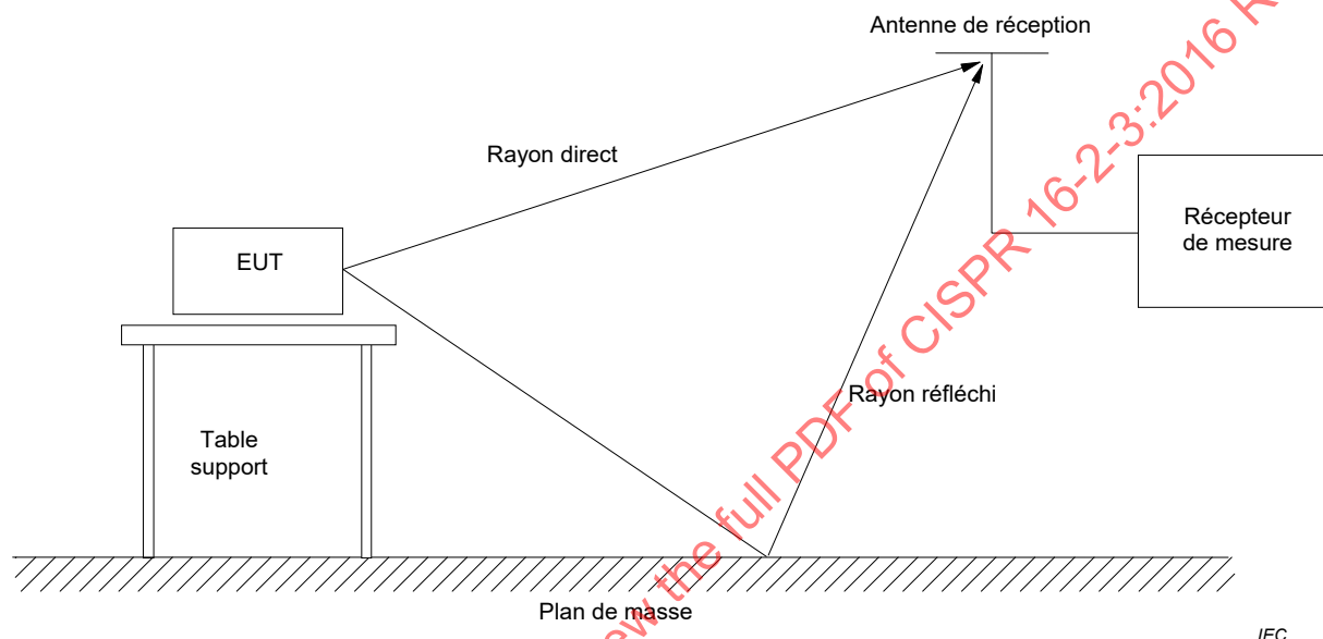
Figure 10 – Concept des mesures de l'amplitude de champ électrique effectués sur un emplacement d'essai en espace libre (OATS) ou dans une chambre semi-anéchoïque (SAC) représentant les rayons directs et réfléchis arrivant sur l'antenne de réception
