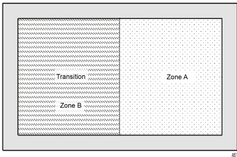
Figure 12 – Essai de hauteur de transition maximale franchissable
