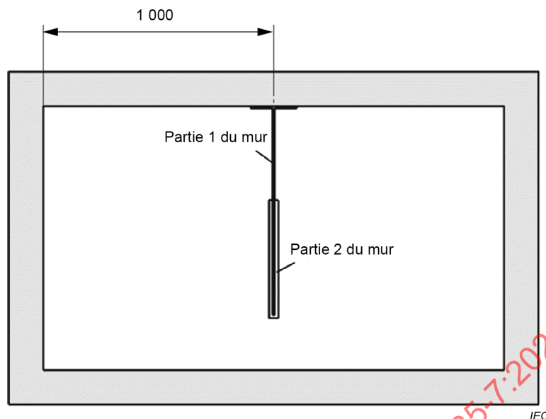
Figure 21 – Banc d'essai avec paroi réglable supplémentaire
