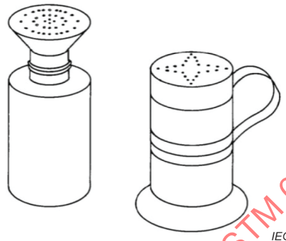
Figure 2 – Dispositifs de distribution de poussière
