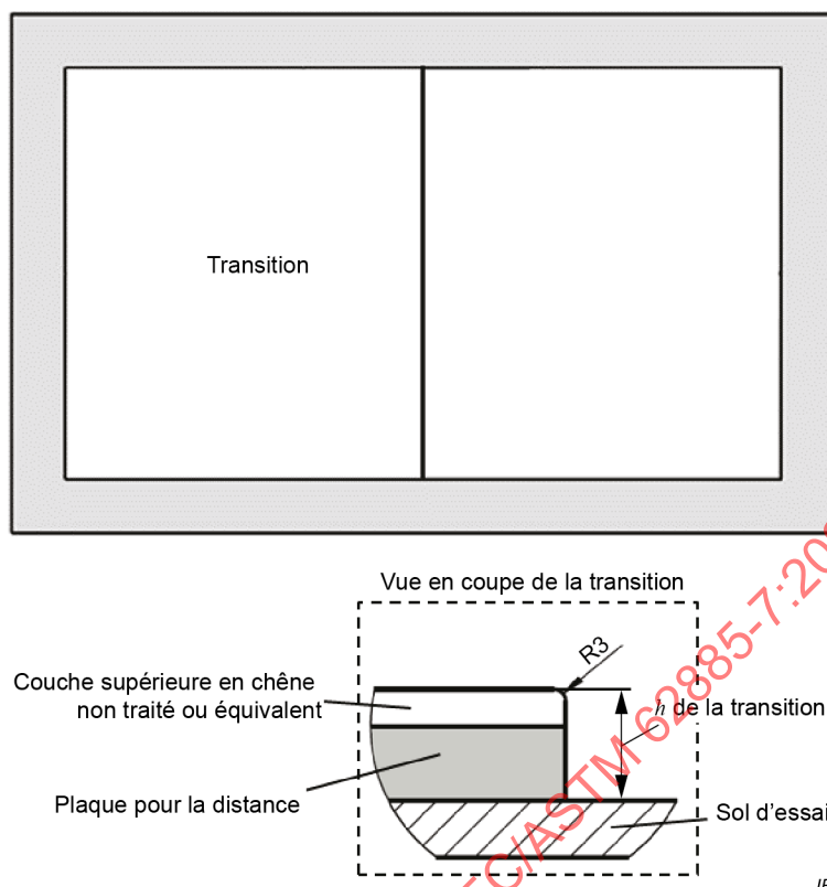
Figure 24 – Banc d’essai avec transition supplémentaire et sa vue en coupe
