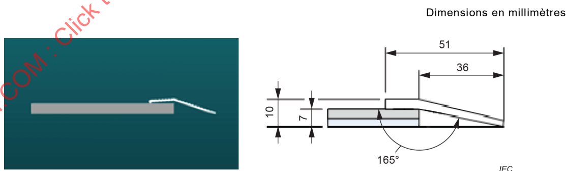
Figure 29 – Représentation de l'installation de la transition métallique
