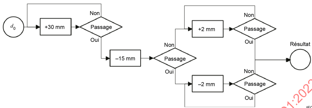
Figure 10 – Processus suggéré pour déterminer la largeur d'écart minimale franchissable
