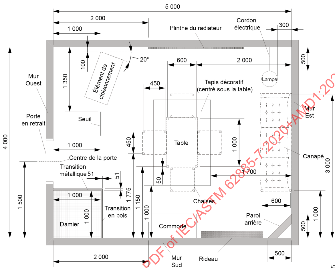
Figure 27 – Configuration du banc d'essai de navigation/couverture
