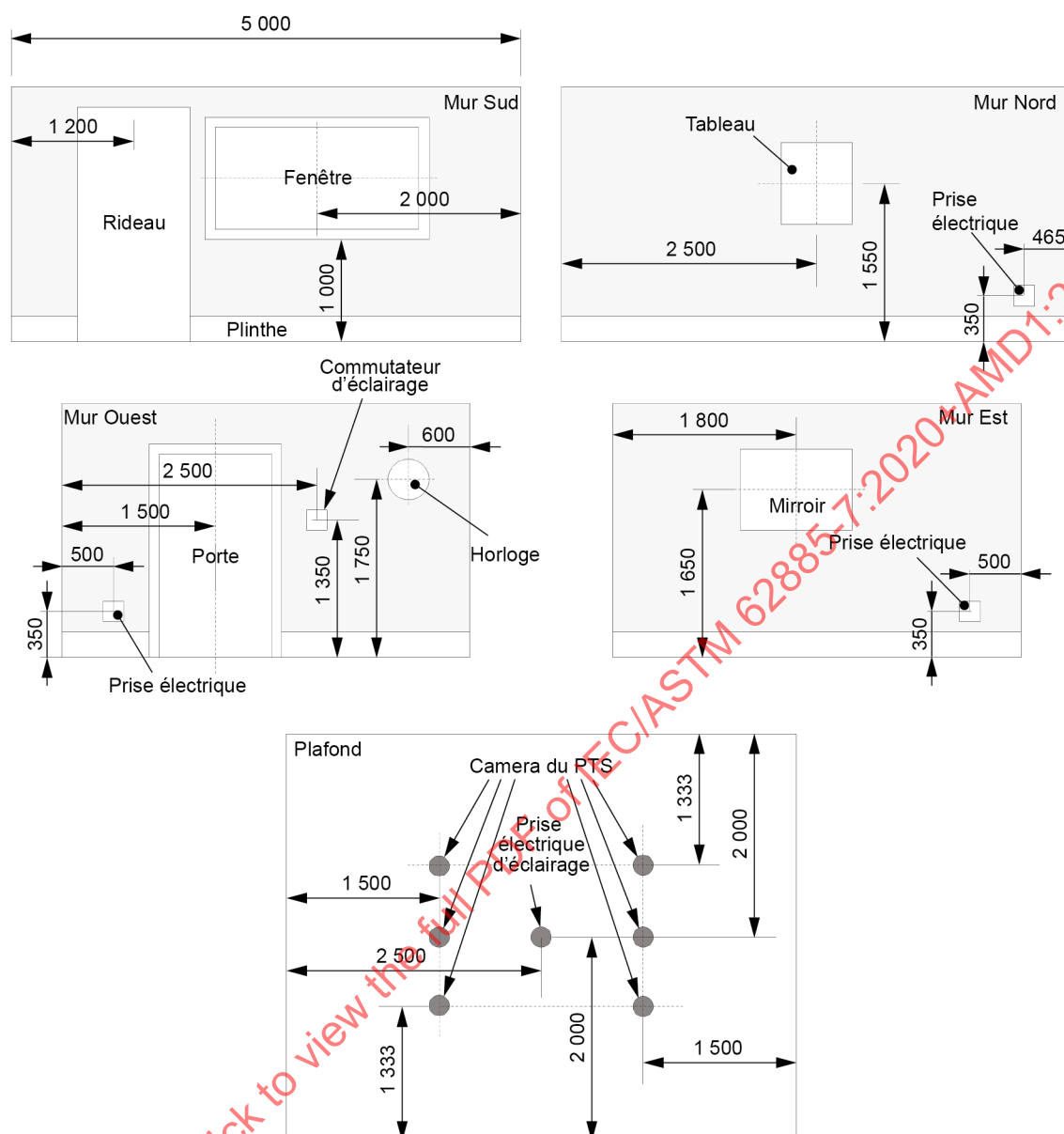
Figure 32 – Configuration des quatre murs et du plafond
