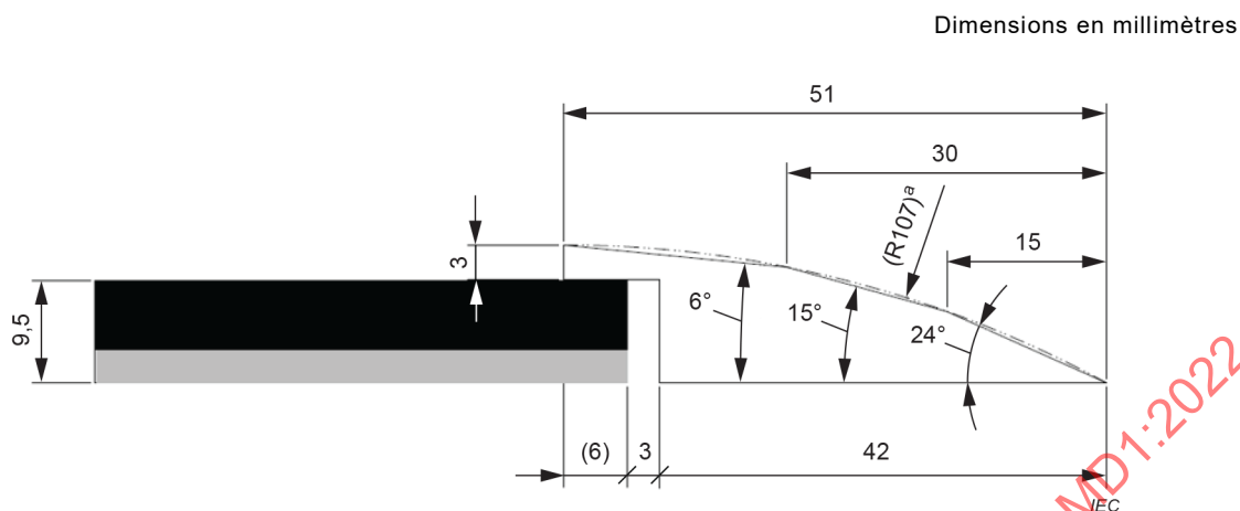
Figure 30 – Représentation de l'installation de la transition en bois
