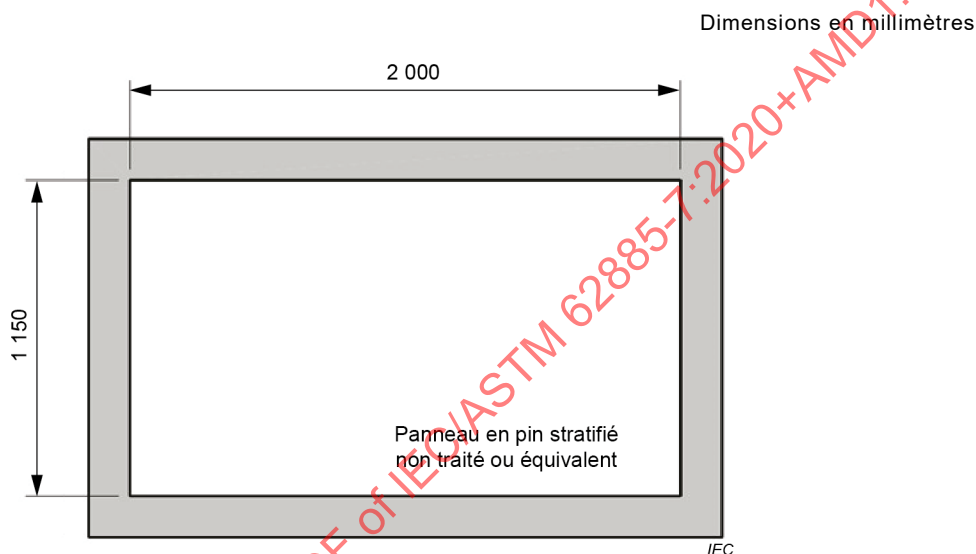
Figure 20 – Configuration du banc d'essai de base pour l'essai de mobilité
