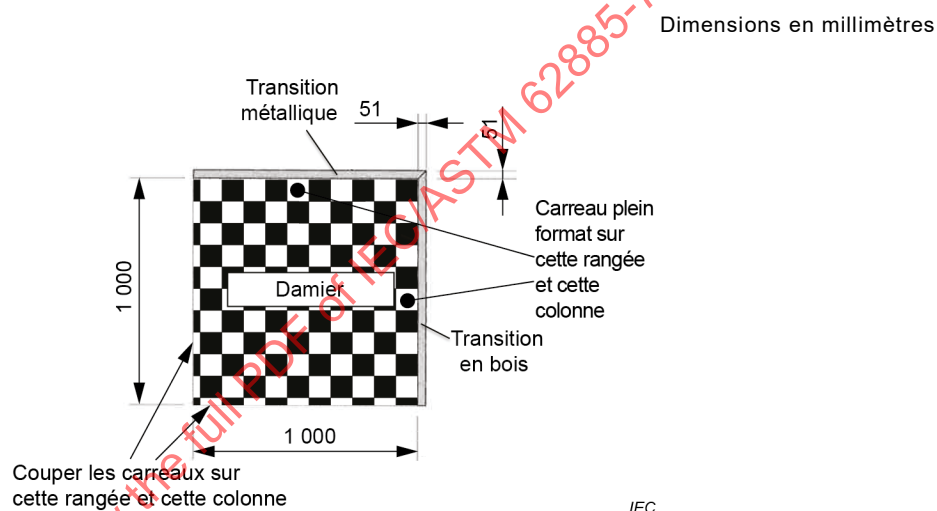
Figure 31 – Vue détaillée du damier et des transitions
