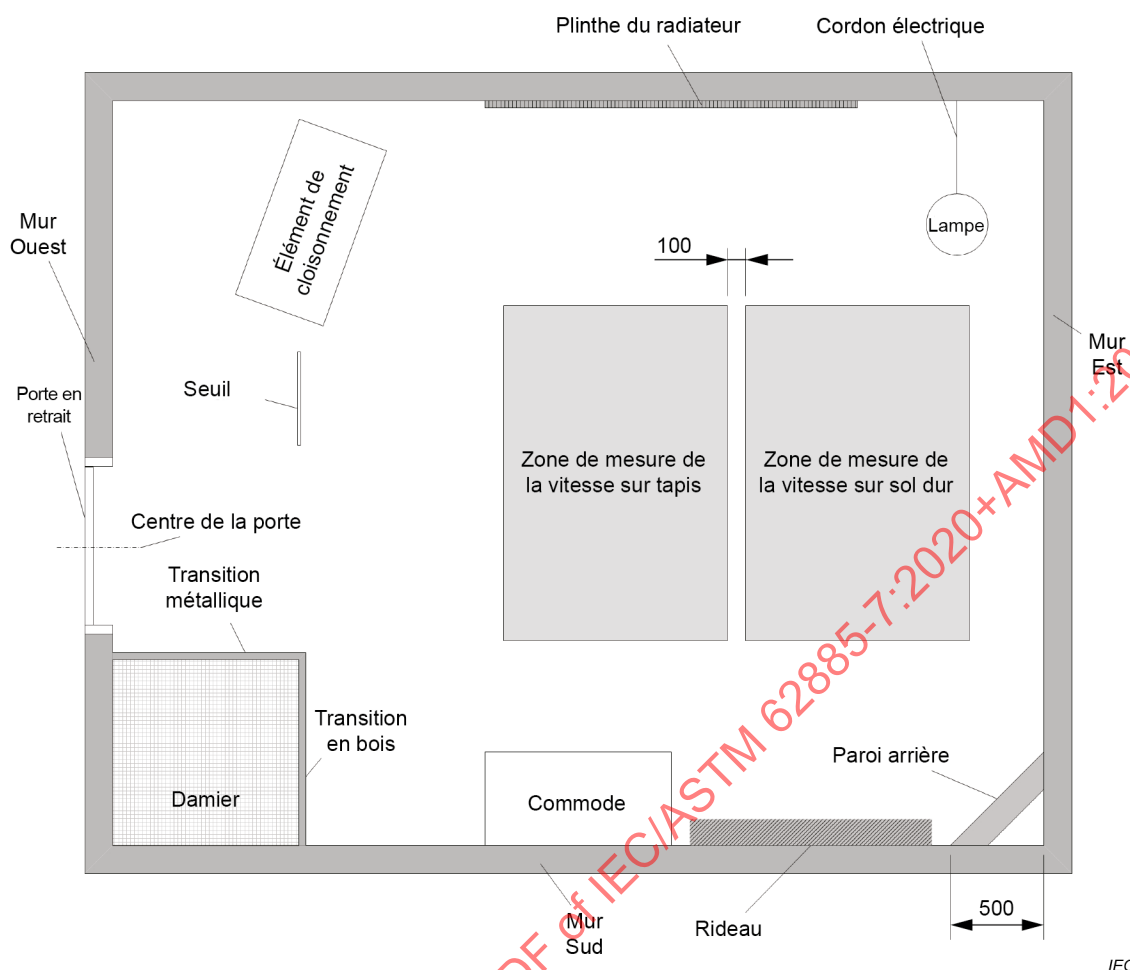
Figure 17 – Zones de mesure de la vitesse en trajectoire rectiligne
