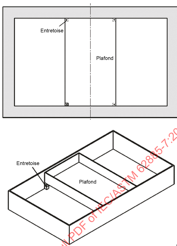
Figure 23 – Banc d’essai avec tunnel supplémentaire
