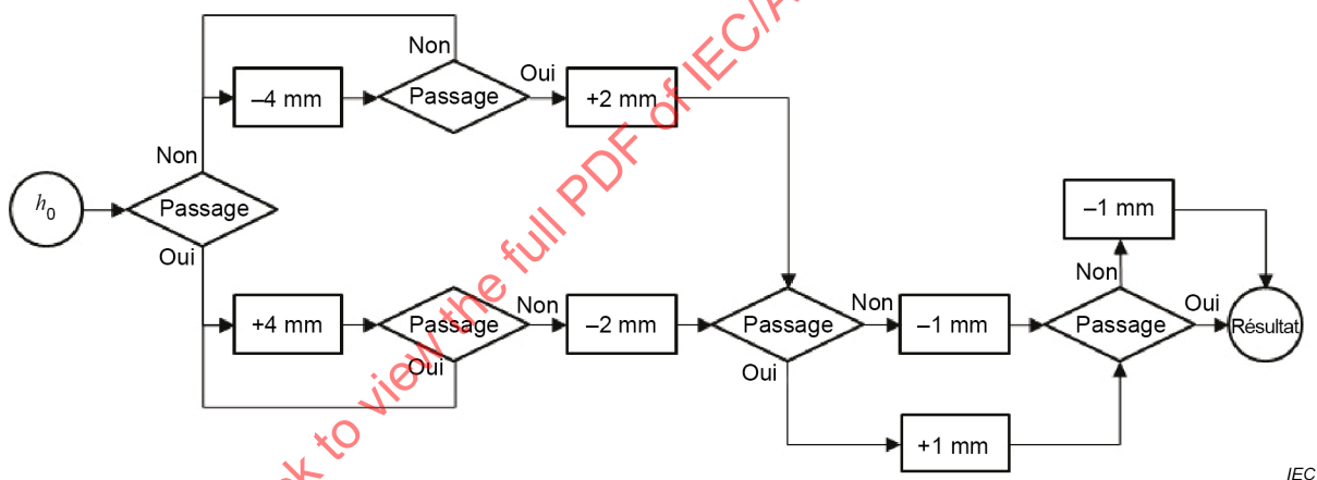
Figure 13 – Processus pour déterminer la hauteur de transition maximale franchissable
