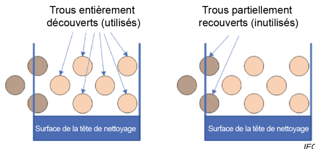
Figure 4 – Alignement des trous du modèle pour grands débris
