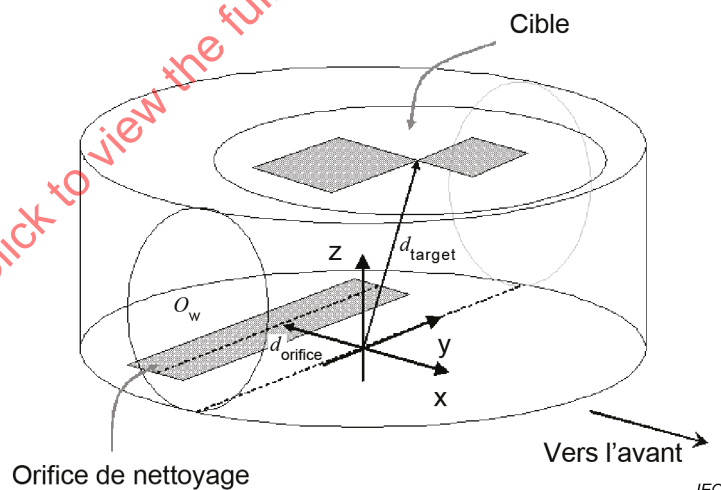
Figure A.1 – Cadre de coordonnées du robot
