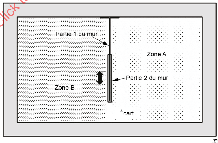
Figure 9 – Essai de largeur d'écart minimale franchissable
