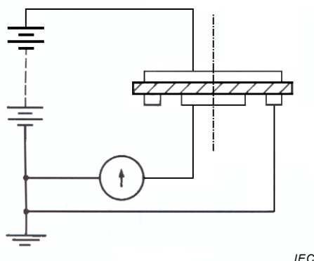
Figure 1 – Connexions de base d'électrodes gardées
