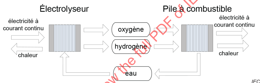
Figure 2 – Schéma d'une entité d'assemblage de cellules/piles PEM réversible séparée
