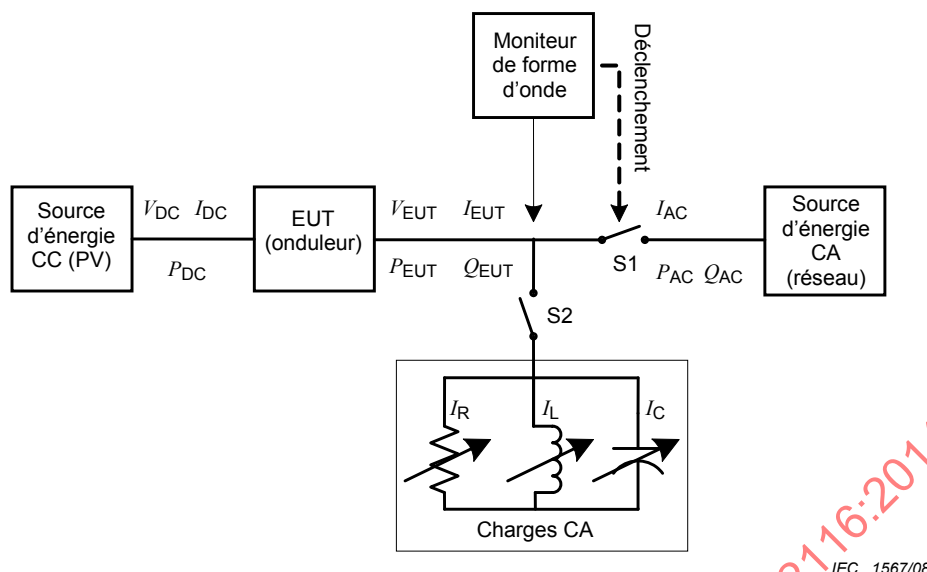
Figure 1 – Circuit d'essai pour la fonction de détection d'ilotage dans un conditionneur de puissance (onduleur)
