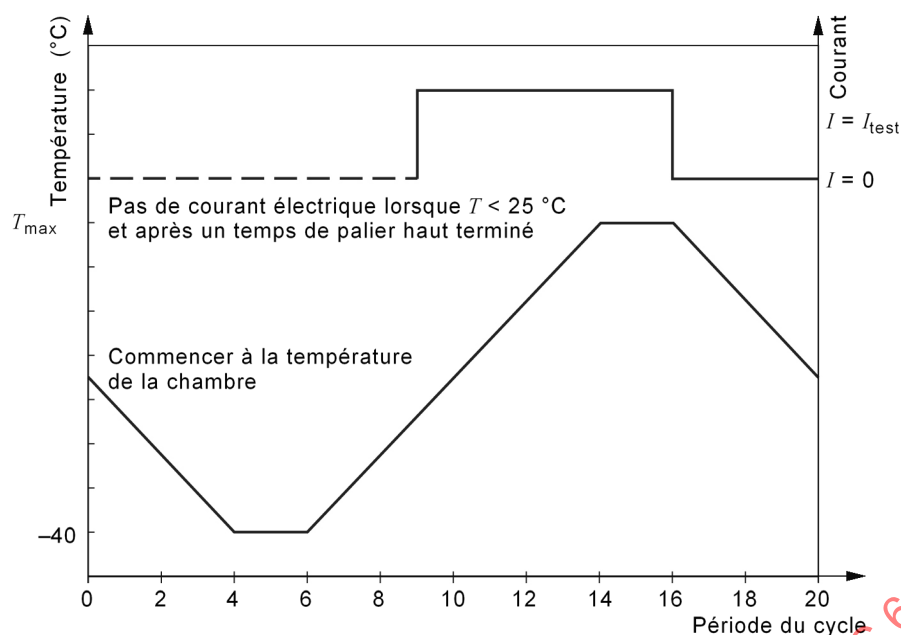
Figure 8 – Profil de température et de courant de l'essai de cyclage thermique (pas à l'échelle)
