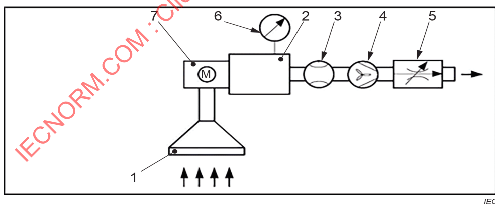
d) Hotte combinée multiple ou extracteur vertical avec ventilateur pour utilisation en extérieur
