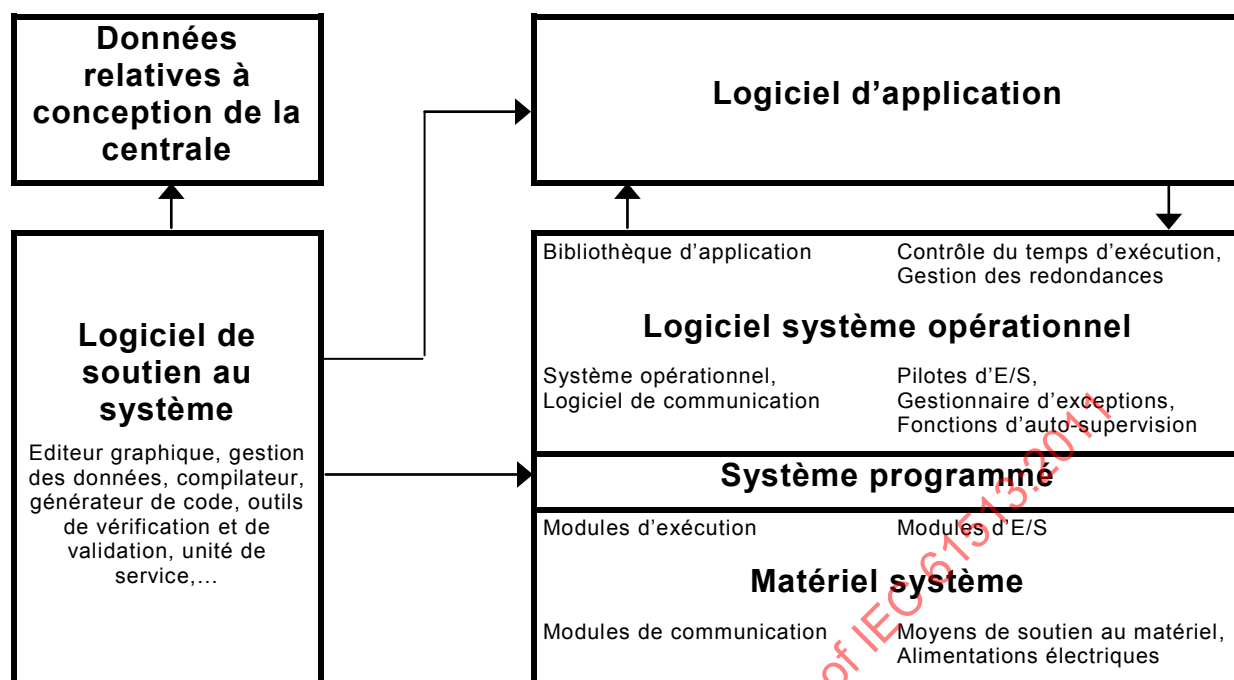
Figure 2 – Relations types entre logiciel et matériel d'un système programmé
