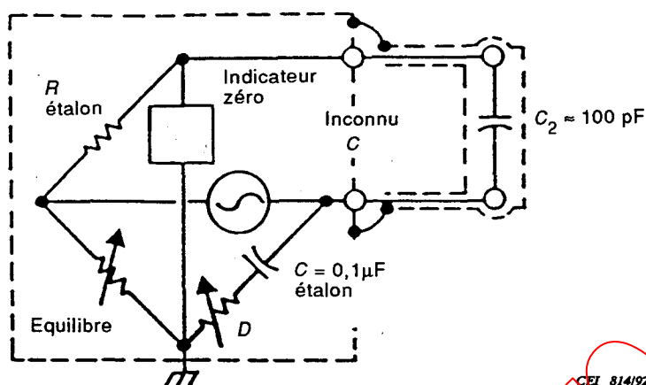
Figure B.2 - Pont de capacité
