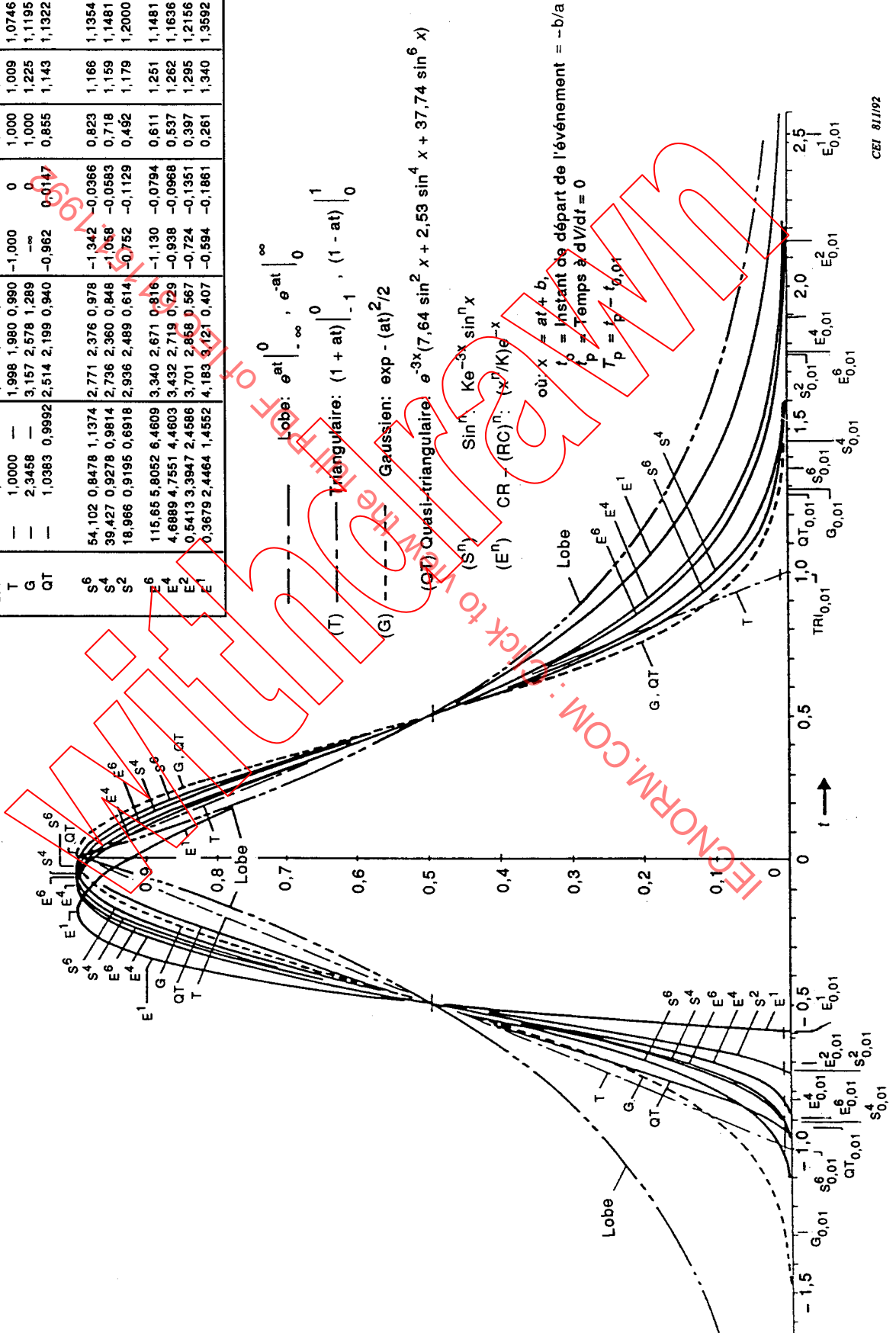
Figure A.2 - Réponse à la fonction échelon des circuits de mise en forme, échelle linéaire
