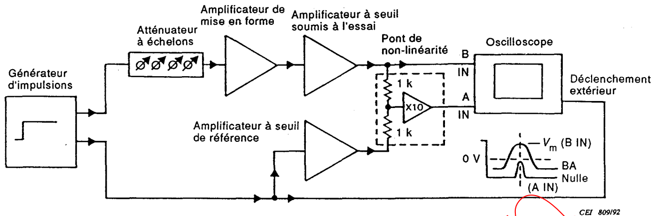
Figure 11 - Montage pour la mesure de la non-linéarité d'un amplificateur à seuil
