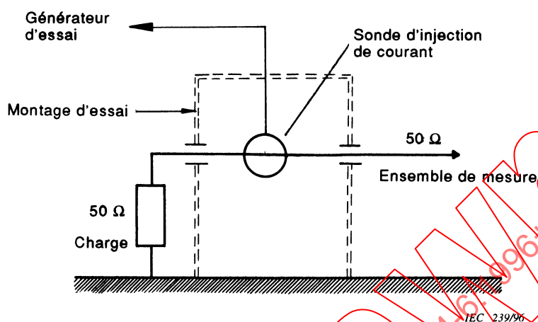
Figure A.1 – Configuration du circuit de réglage du niveau sur un montage d'essai 50 \Omega
