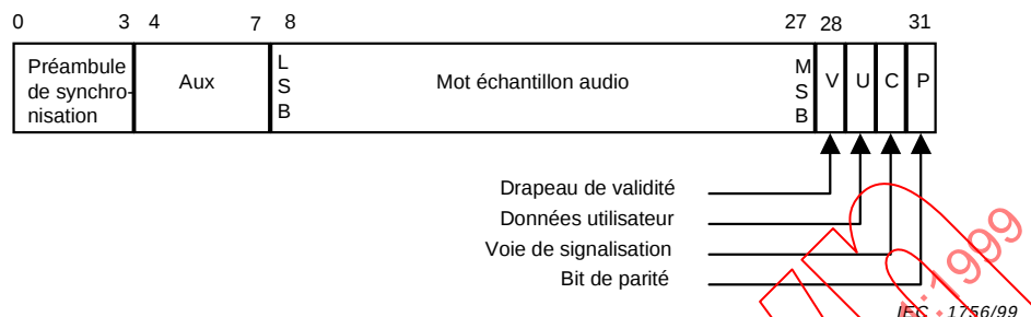
Figure 1 – Format de la sous-trame (application linéaire MIC)
