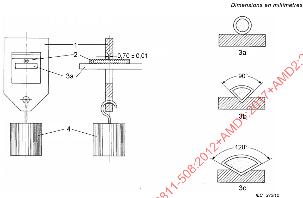
Légende 1 étrier d'essai 3a, 3b, 3c supports 2 échantillon 4 charge Figure 1 – Dispositif d'empreinte
