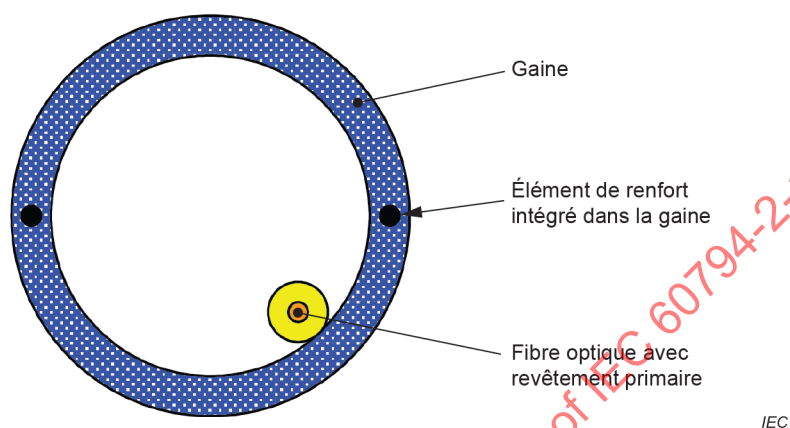
Figure A.1 – Câble simplex à fibres optiques sans revêtement protecteur à structure lâche
