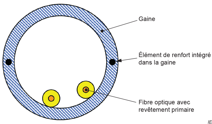
Figure A.3 – Câble duplex à fibres optiques sans revêtement protecteur à structure lâche
