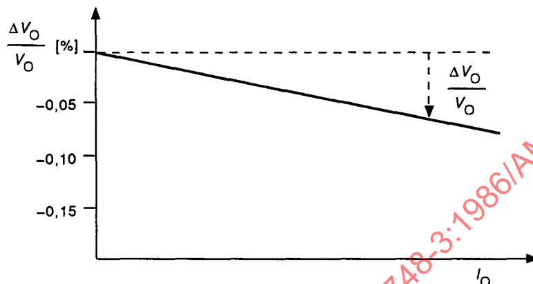
Figure 54 – Courbe de régulation de la charge \Delta V_O/V_O en fonction du courant de sortie I_O
