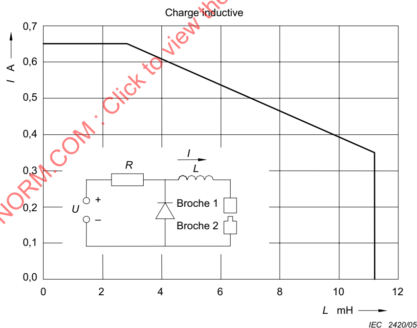
Figure 37 – Courant maximal admissible I en fonction de l'inductance L mesurée dans un circuit inductif dans un ENVIRONNEMENT RICHE EN OXYGÈNE (voir 11.2.2.1)
