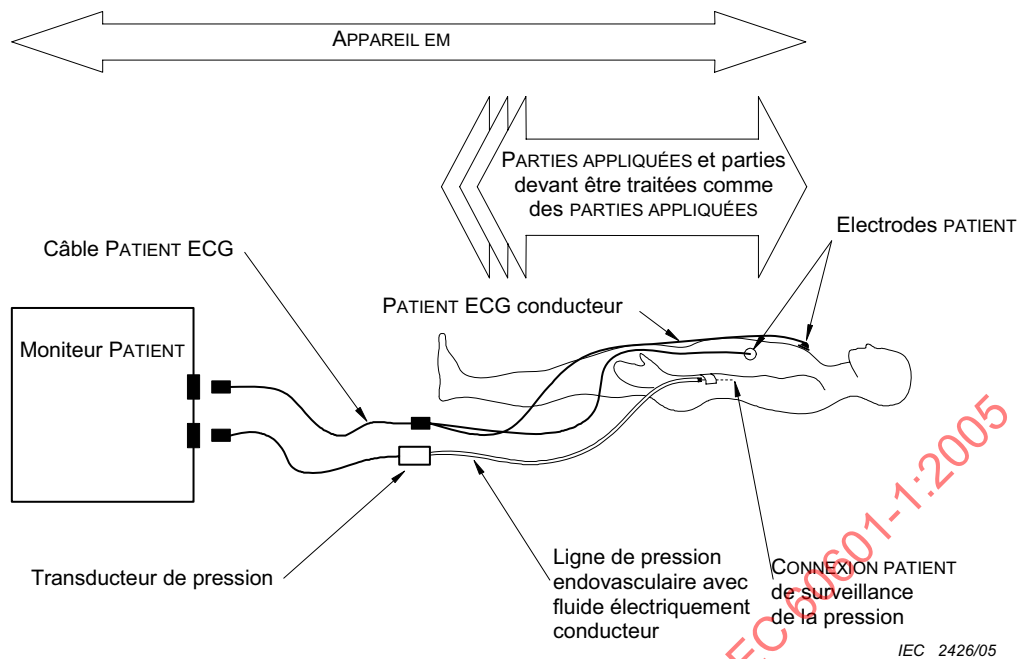
Figure A.4 – Identification de l'APPAREIL EM, DES PARTIES APPLIQUÉES et des CONNEXIONS PATIENT dans un moniteur PATIENT multifonctions avec dispositifs de surveillance endovasculaire de la pression
