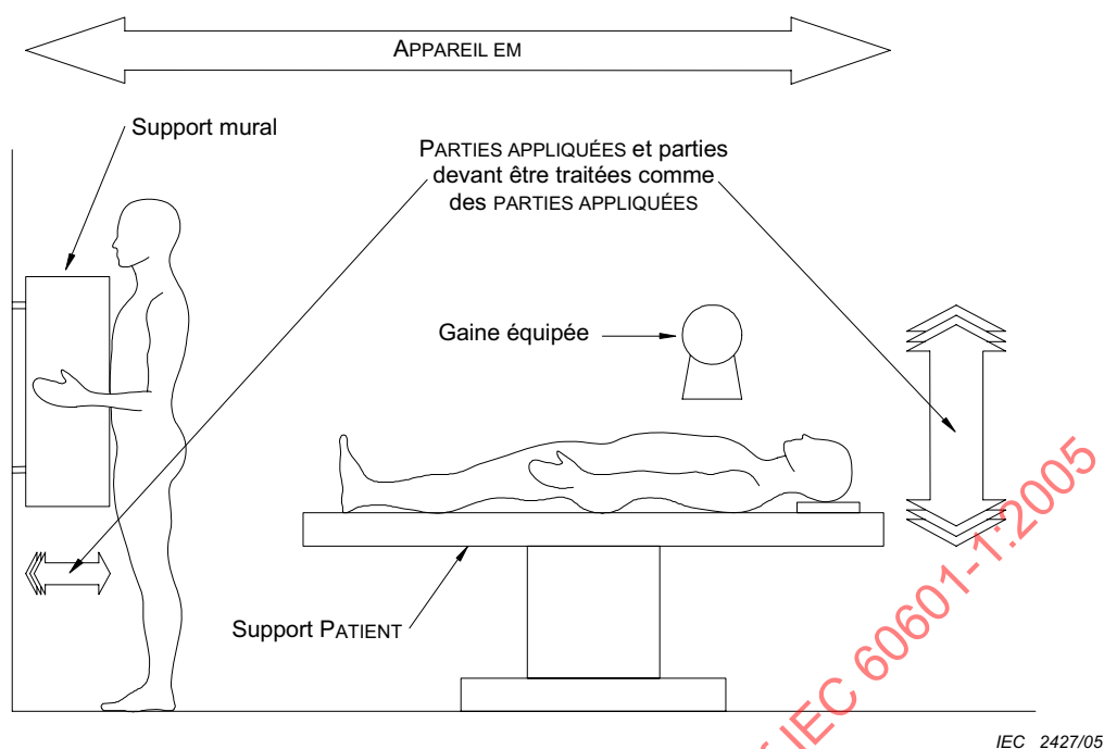
Figure A.5 – Identification des PARTIES APPLIQUÉES et des CONNEXIONS PATIENT dans un SYSTÈME EM À RAYONS X
