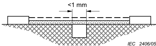
Figure 22 – LIGNE DE FUITE et DISTANCE DANS L'AIR – Exemple 1
