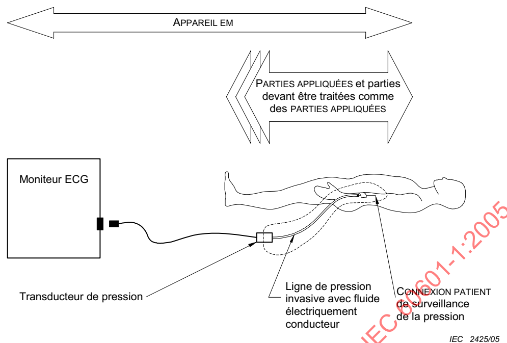
Figure A.3 – Identification de l'APPAREIL EM, DES PARTIES APPLIQUÉES et des CONNEXIONS PATIENT dans un moniteur PATIENT avec dispositifs de surveillance endovasculaire de la pression
