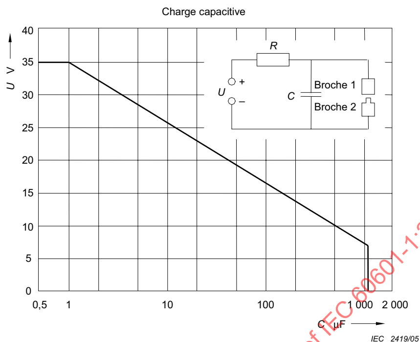
Figure 36 – Tension maximale admissible U en fonction de la capacité C mesurée dans un circuit capacitif utilisé dans un ENVIRONNEMENT RICHE EN OXYGÈNE (voir 11.2.2.1)
