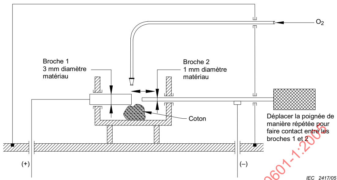
Figure 34 – Appareillage d'essai d'inflammation par étincelles (voir 11.2.2.1)
