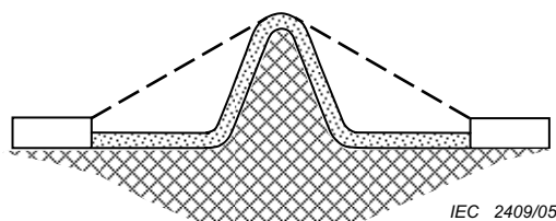
Figure 26 – LIGNE DE FUITE et DISTANCE DANS L'AIR – Exemple 5
