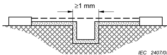
Figure 23 – LIGNE DE FUITE et DISTANCE DANS L'AIR – Exemple 2
