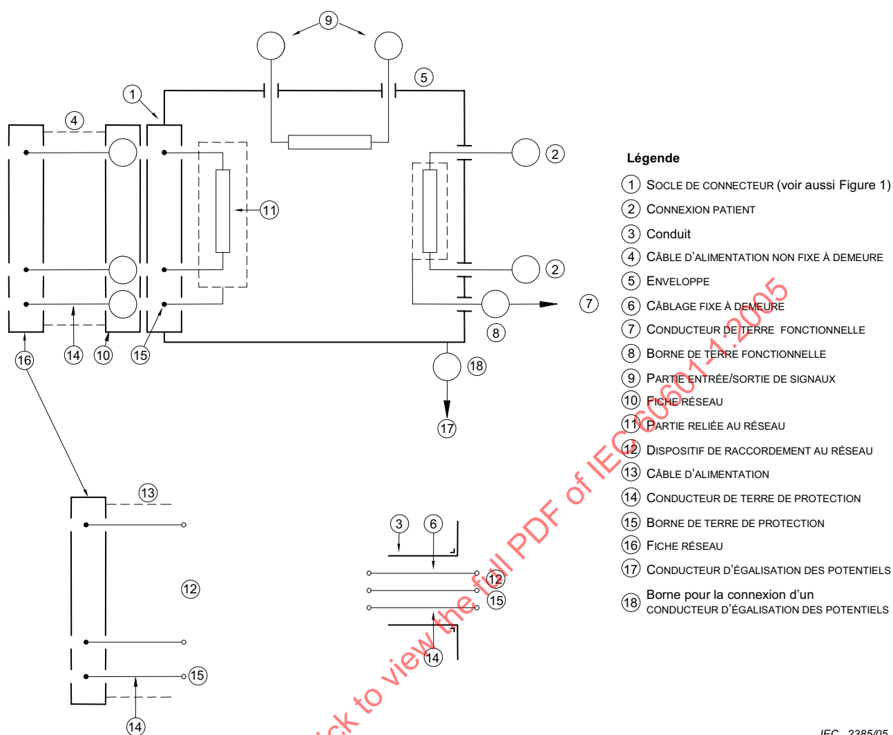
Figure 2 – Exemple de bornes et conducteurs définis (voir définitions)
