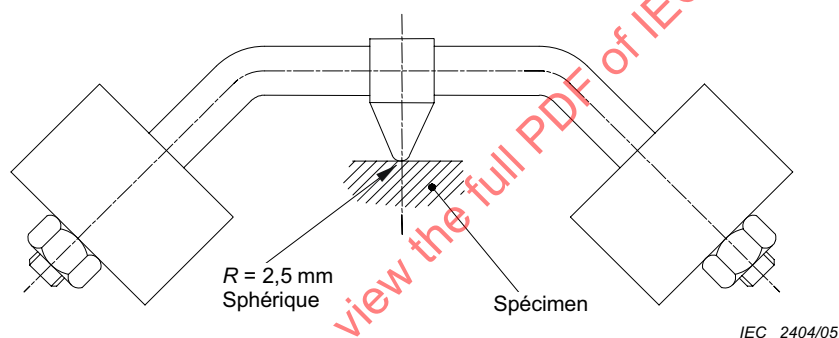
Figure 21 – Appareillage pour l'essai à la bille (voir 8.8.4.1)
