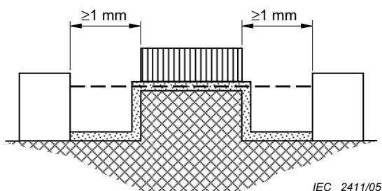
Figure 28 – LIGNE DE FUITE et DISTANCE DANS L'AIR – Exemple 7
