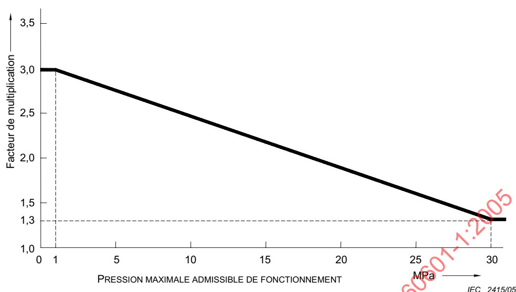
Figure 32 – Rapport entre la PRESSION D'ESSAI HYDRAULIQUE et la PRESSION MAXIMALE ADMISSIBLE DE FONCTIONNEMENT (voir 9.7.5)
