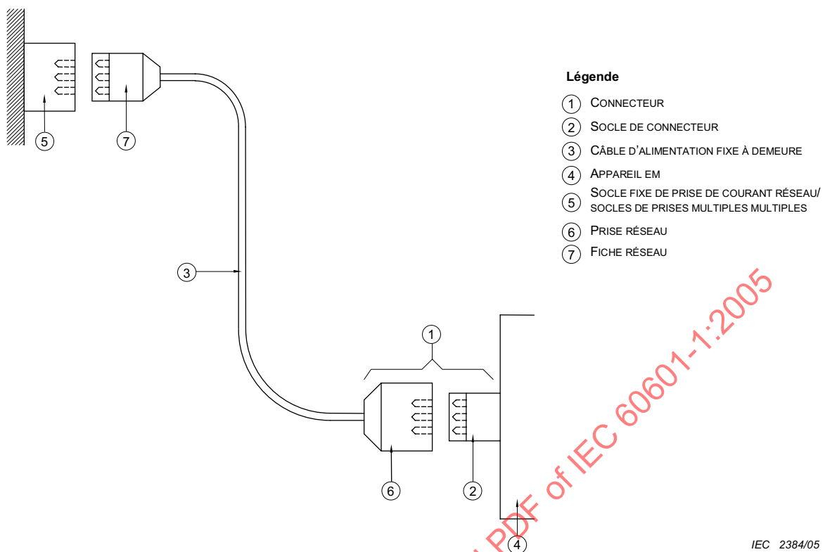
Figure 1 – Raccordement au réseau non fixé à demeure (voir définitions)
