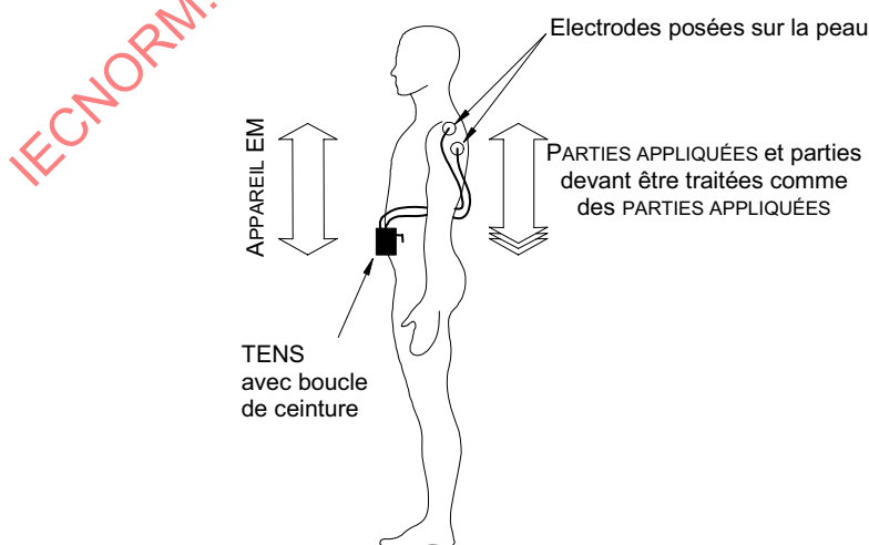
Figure A.6 – Identification de l'APPAREIL EM, des PARTIES APPLIQUÉES et des CONNEXIONS PATIENT dans un neurostimulateur électrique transcutané (TENS) destiné à être porté sur la ceinture du PATIENT et connecté à des électrodes sur le haut du bras du PATIENT
