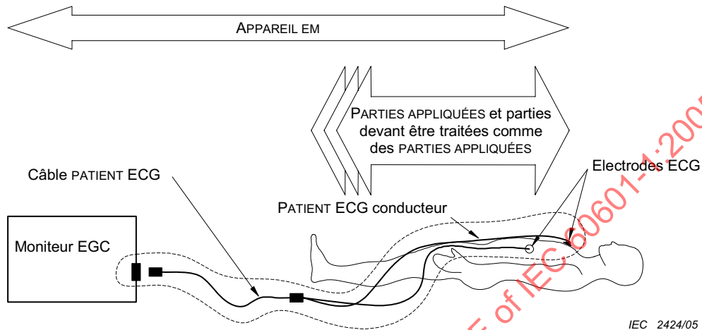
Figure A.2 – Exemple d'isolation d'une PARTIE APPLIQUÉE DE TYPE F avec isolation incorporée dans l'APPAREIL EM
