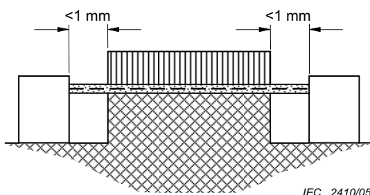
Figure 27 – LIGNE DE FUITE et DISTANCE DANS L'AIR – Exemple 6
