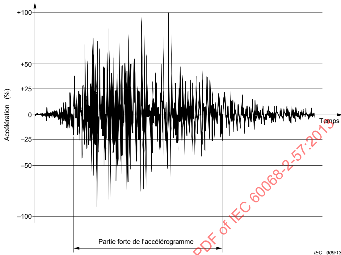
Figure 3 – Accélérogramme caractéristique
